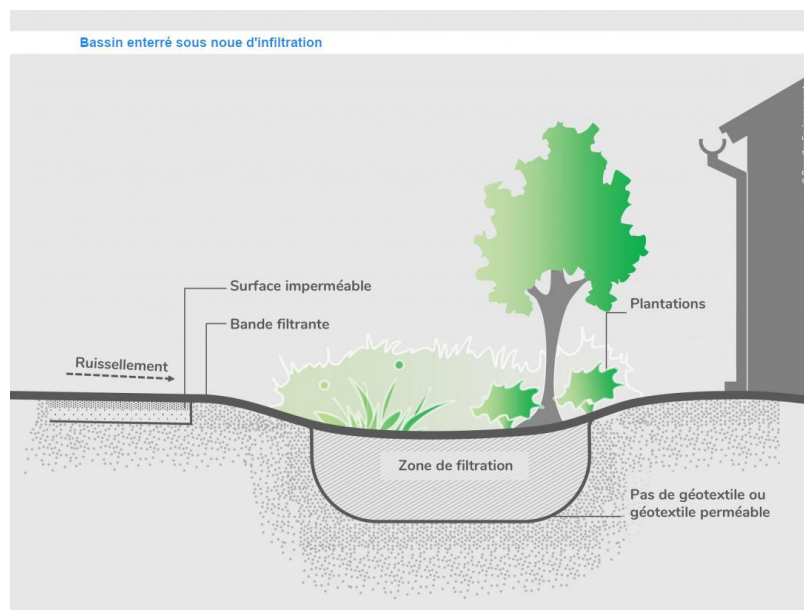
Figure 13 : Coupe de principe d'un bassin sous noue d'infiltration
