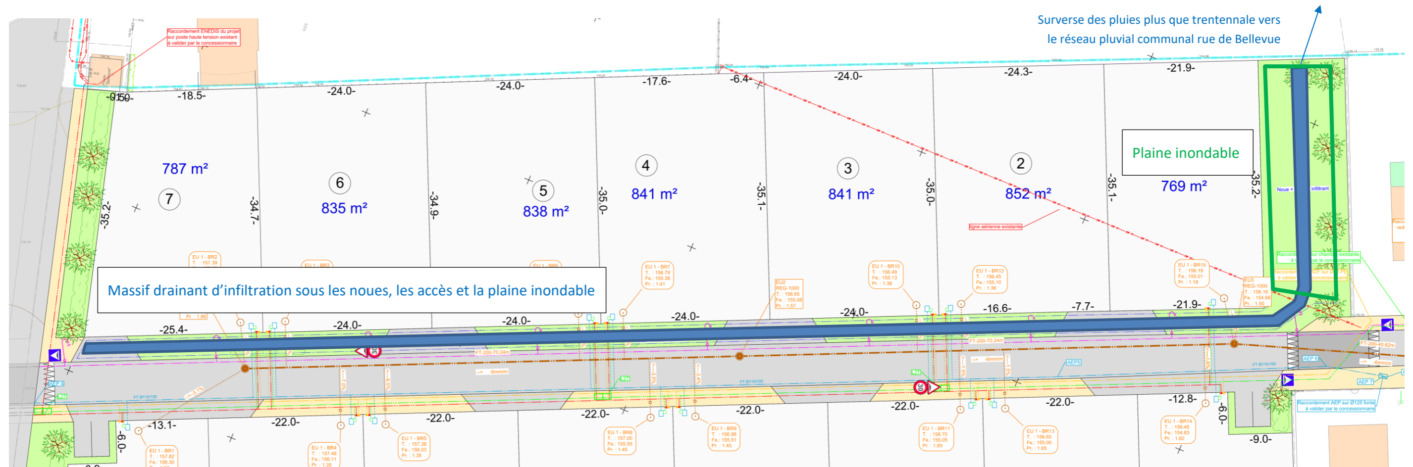
Figure 11 : Plan de gestion des eaux pluviales
