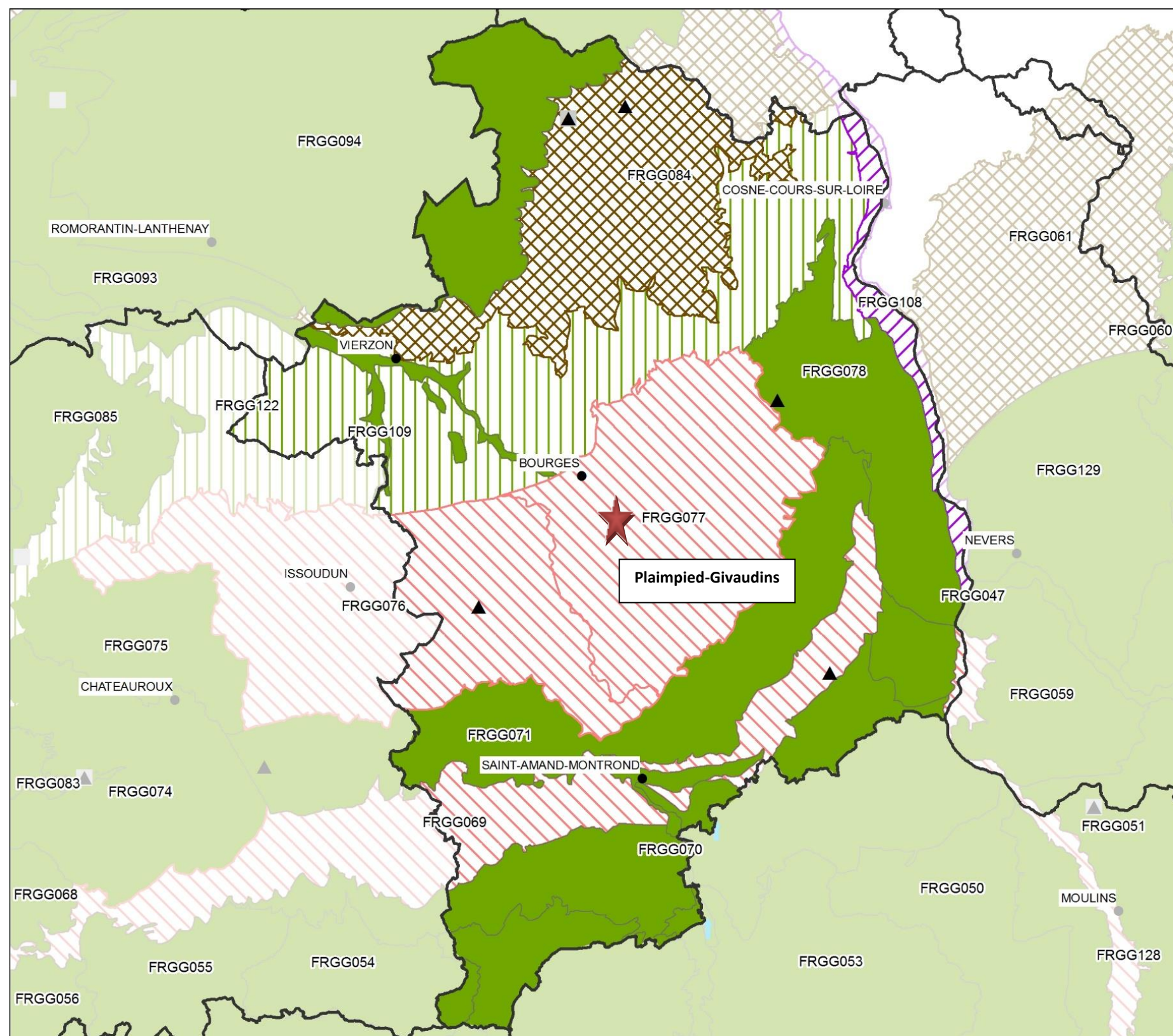
Figure 20 : Carte de l'état chimique des masses d'eau souterraines. (Source : BRGM, eaufrance)
